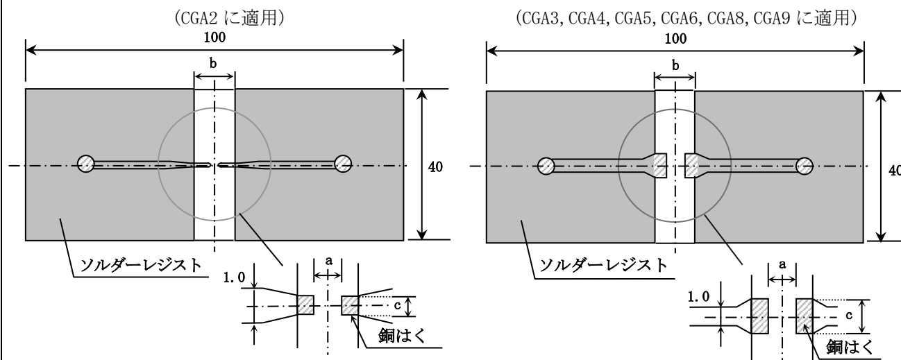
付図－２ プリント基板設計図
