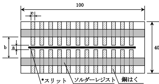
付図－２ プリント基板設計図
