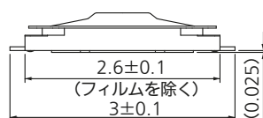
C-C断面図
