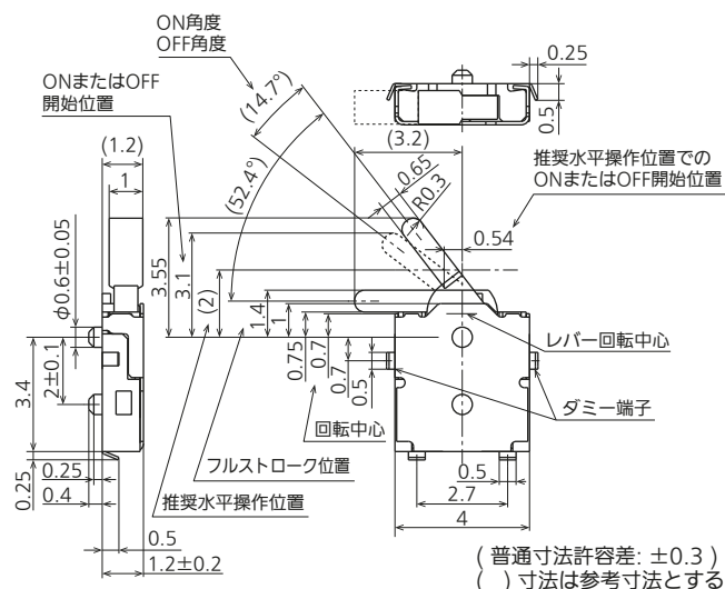
外形寸法図
