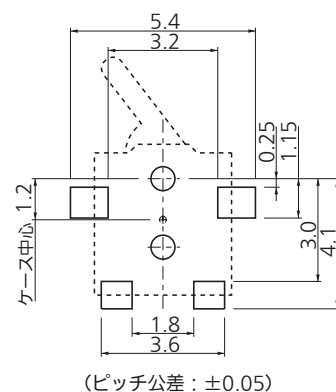
プリント基板取付穴参考図
