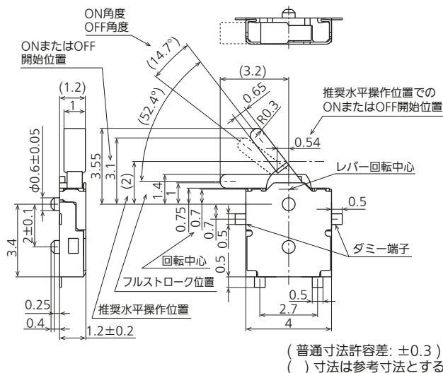
外形寸法図
