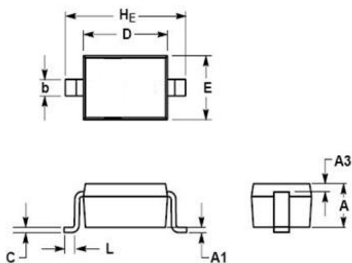
SOD323
