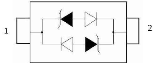
SOD323
