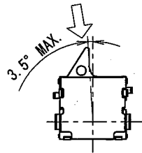
FIG1 TOLERANCE ANGLE WHEN VERTICALLY OPERATING. 垂直動作時 許容角度
