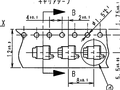
④ CARRIER TAPE キャリアテープ
