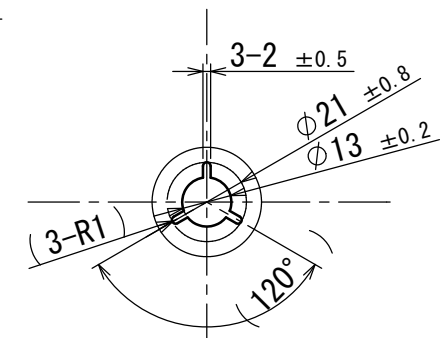
DETAIL OF A 詳細図 A
