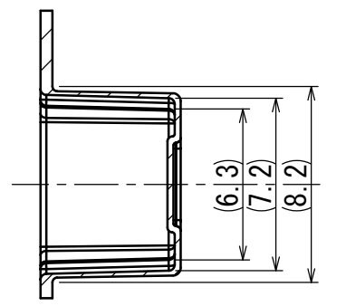
断面図 B-B
