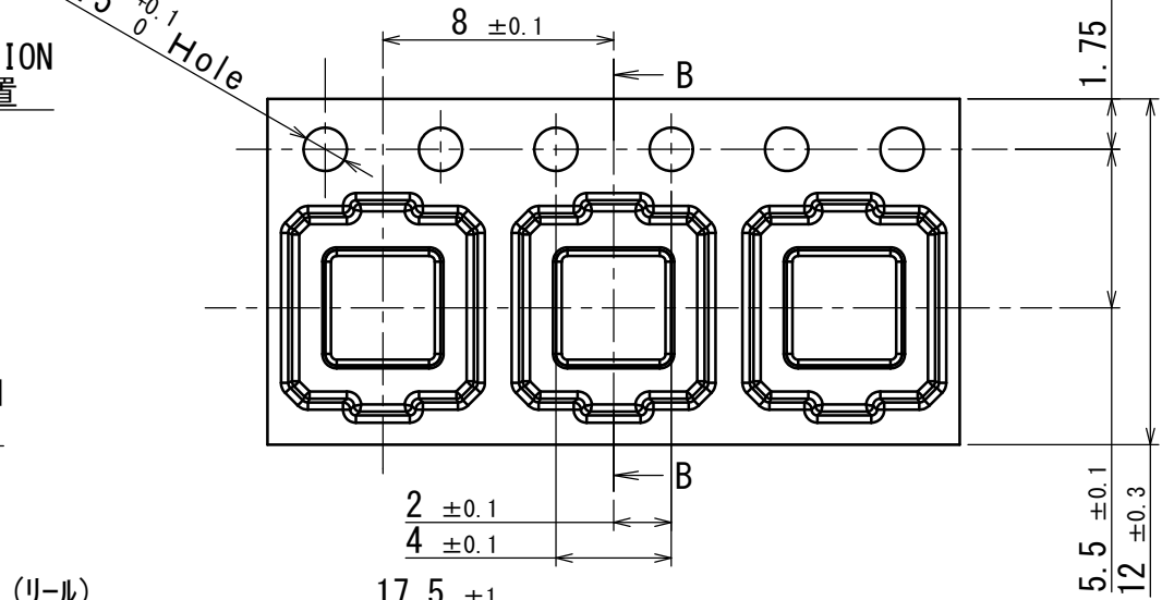
CARRIER TAPE (キャリアテープ)
