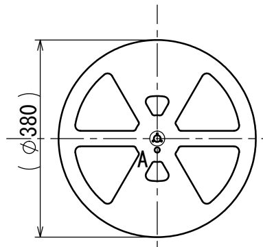
REEL (リール)
