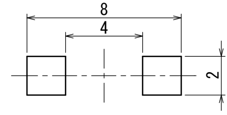
PWB LAND DEMENSIONS プリント基板ランド寸法
