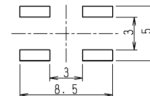
b) DIMENSION FOR REFLOW SOLDERING リフロー半田用ハ°ターン図
