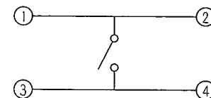
回路図 CIRCUIT DIAGRAM
