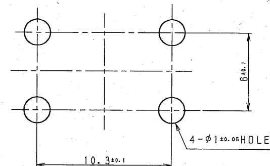
プリント基盤取付穴寸法 (スイッチ取付面側より見る) P.C BOARD MOUNTING HOLE DIMENSIONS (WHEN VIEWED FROM SWITCH MOUNTING FACE)
