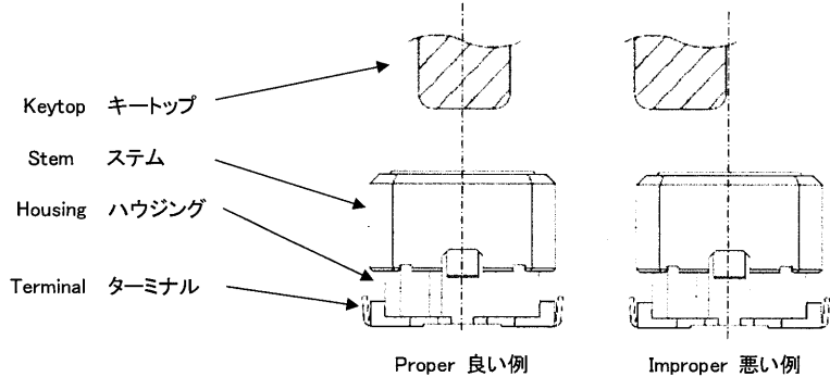
Fig 2: Keytop and Stem 図 2: キートップとステムの関係
