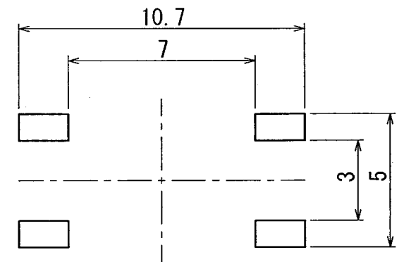
PRINTED CIRCUIT BOARD LAND DIMENSION プリント基板推奨ランド寸法 (5:1) (WHEN VIEWED FROM THE SWITCH MOUNTING FACE) (スイッチ取り付け面より見る)
