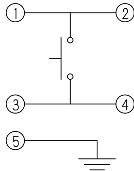
回路図 CIRCUIT DIAGRAM
