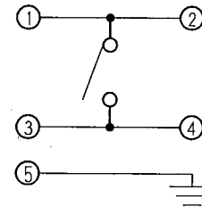
回路図 CIRCUIT DIAGRAM
