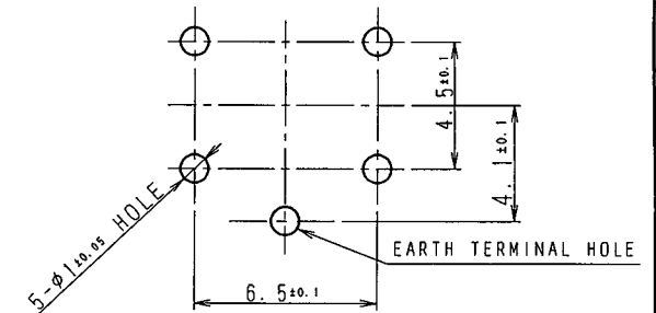
プリント基盤取付穴寸法 (スイッチ取付面側より見る) P.C BOARD MOUNTING HOLE DIMENSIONS (WHEN VIEWED FROM SWITCH MOUNTING FACE)
