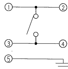
回路図 CIRCUIT DIAGRAM
