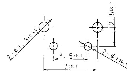
プリント基板取付穴寸法 (スイッチ取付面側より見る) P.C BOARD MOUNTING HOLE DIMENSIONS (WHEN VIEWED FROM SWITCH MOUNTING FACE)
