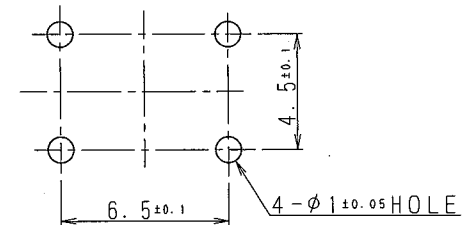
プリント基板取付寸法 (スイッチ取付面側より見る) P.C BOARD MOUNTING HOLE DIMENSIONS (WHEN VIEWED FROM SWITCH MOUNTING FACE)
