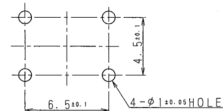
プリント基盤取付穴寸法 (スイッチ取付面側より見る) P.C BOARD MOUNTING HOLE DIMENSIONS (WHEN VIEWED FROM SWITCH MOUNTING FACE)
