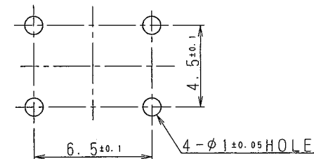
プリント基盤取付寸法 (スイッチ取付面側より見る) P.C BOARD MOUNTING HOLE DIMENSIONS (WHEN VIEWED FROM SWITCH MOUNTING FACE)
