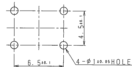
プリント基盤取付穴寸法 (スイッチ取付面側より見る) P.C BOARD MOUNTING HOLE DIMENSIONS (WHEN VIEWED FROM SWITCH MOUNTING FACE)
