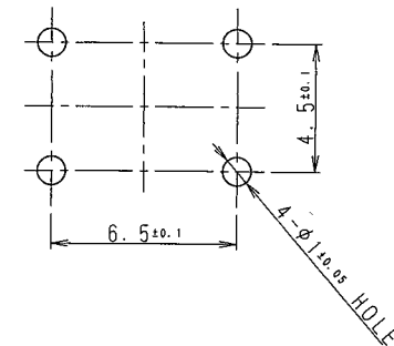
プリント基盤取付穴寸法 (スイッチ取付面側より見る) P.C BOARD MOUNTING HOLE DIMENSIONS (WHEN VIEWED FROM SWITCH MOUNTING FACE)
