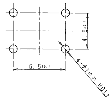
プリント基盤取付穴寸法 (スイッチ取付面側より見る) P.C BOARD MOUNTING HOLE DIMENSIONS (WHEN VIEWED FROM SWITCH MOUNTING FACE)
