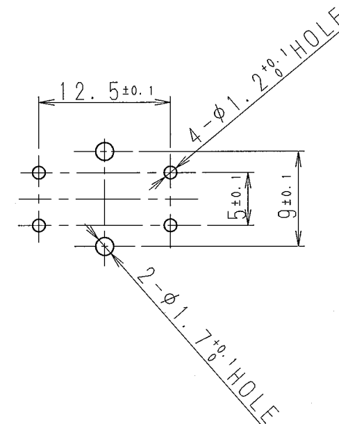
プリント基盤取付穴寸法 (スイッチ取付面側より見る) P.C BOARD MOUNTING HOLE DIMENSIONS (WHEN VIEWED FROM SWITCH MOUNTING FACE)
