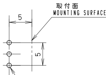
端子取付穴寸法図 (挿入側より見た図) (許容差±0.1)
