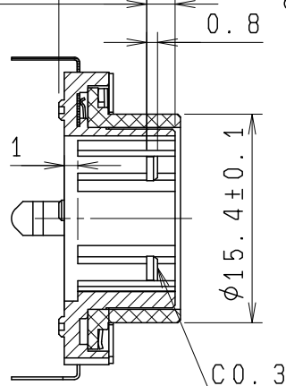
断面YY SECTION YY
